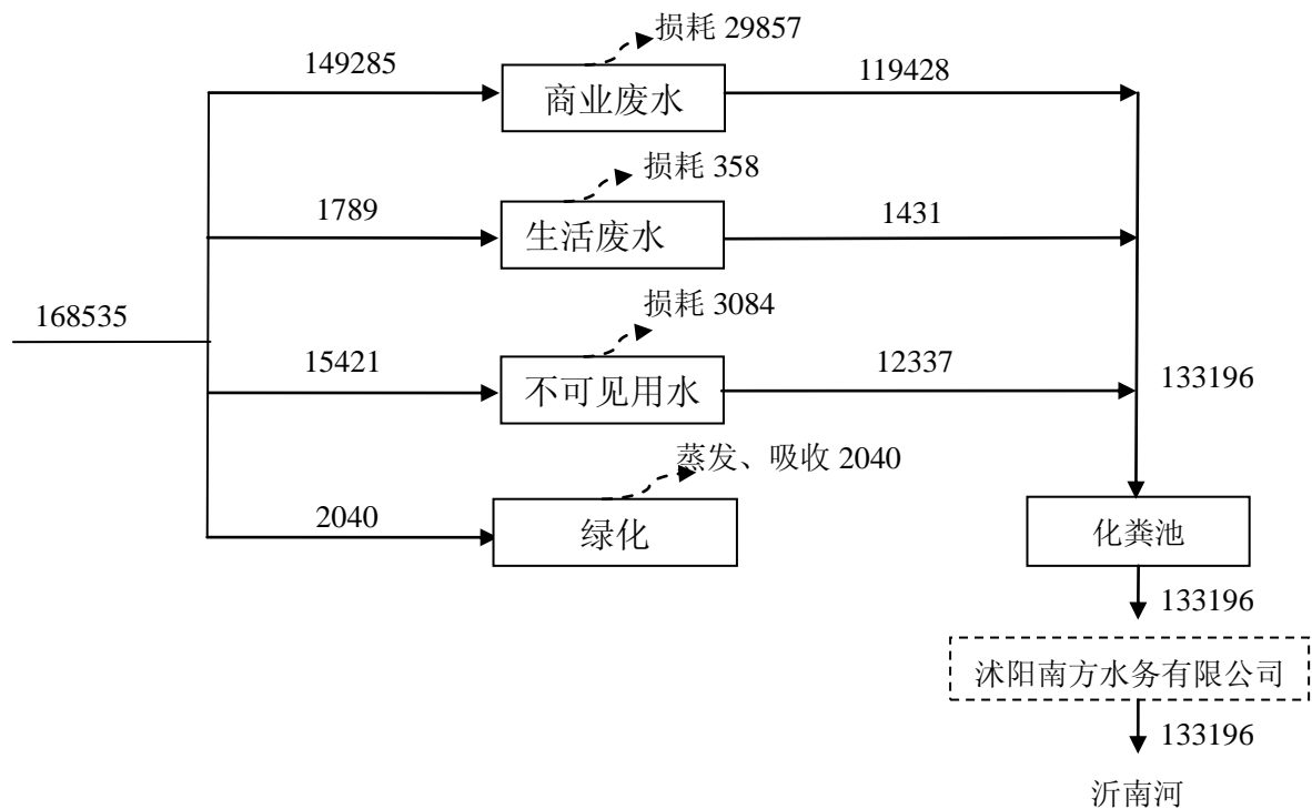
图 5-1 建设项目水平衡图 (t/a)
