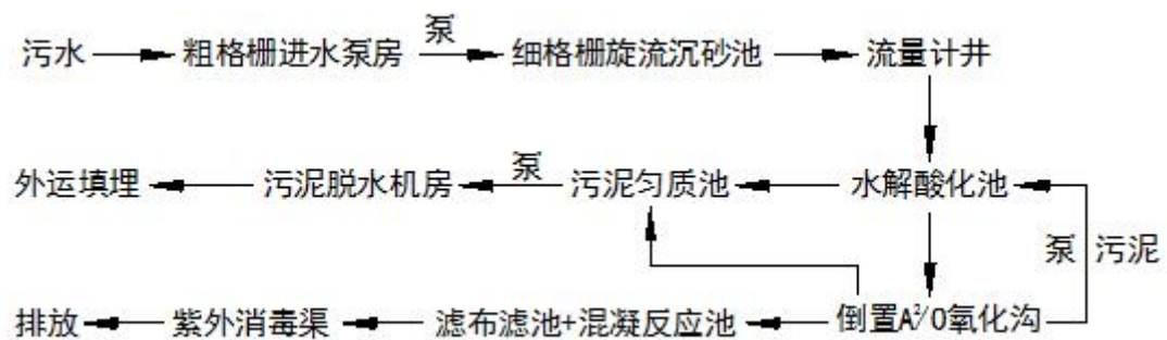
图 6-1 金风环保（沭阳）有限公司污水处理工艺流程图
