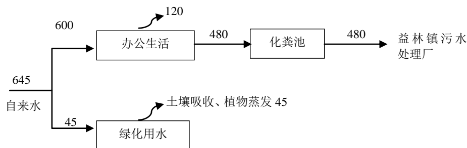
图 5-3 本项目总用水量平衡图 (t/a)
