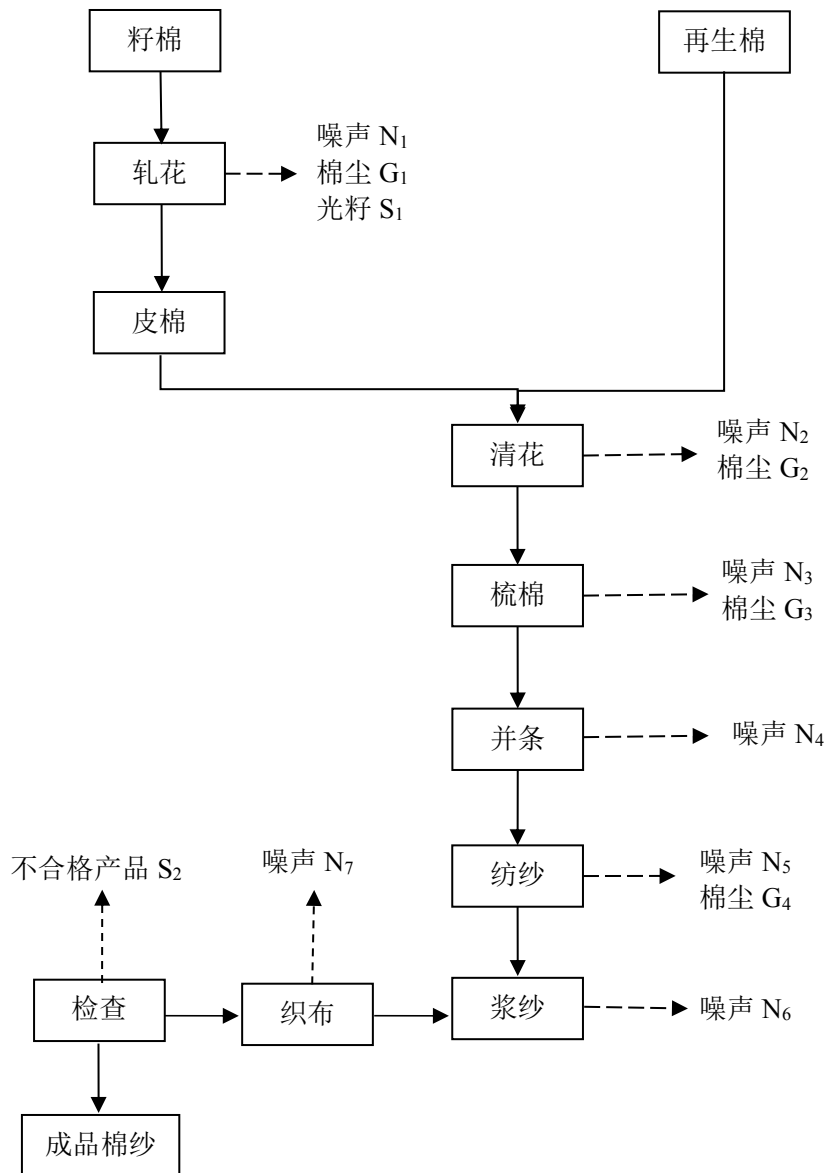
图 5-1 项目棉布加工工艺及主要产污环节图
