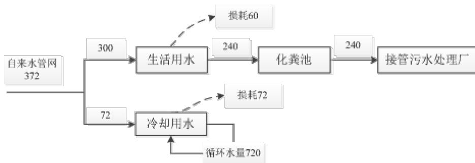
图 5-2 建设项目水平衡图 (t/a)
