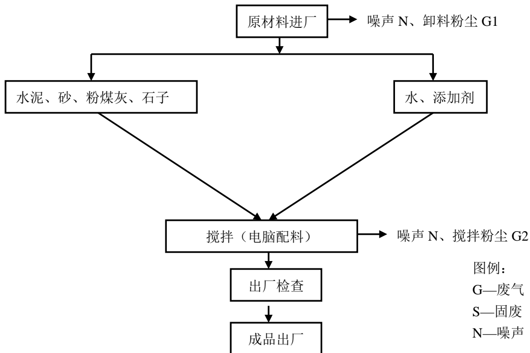
图 5-1 营运期生产工艺流程
