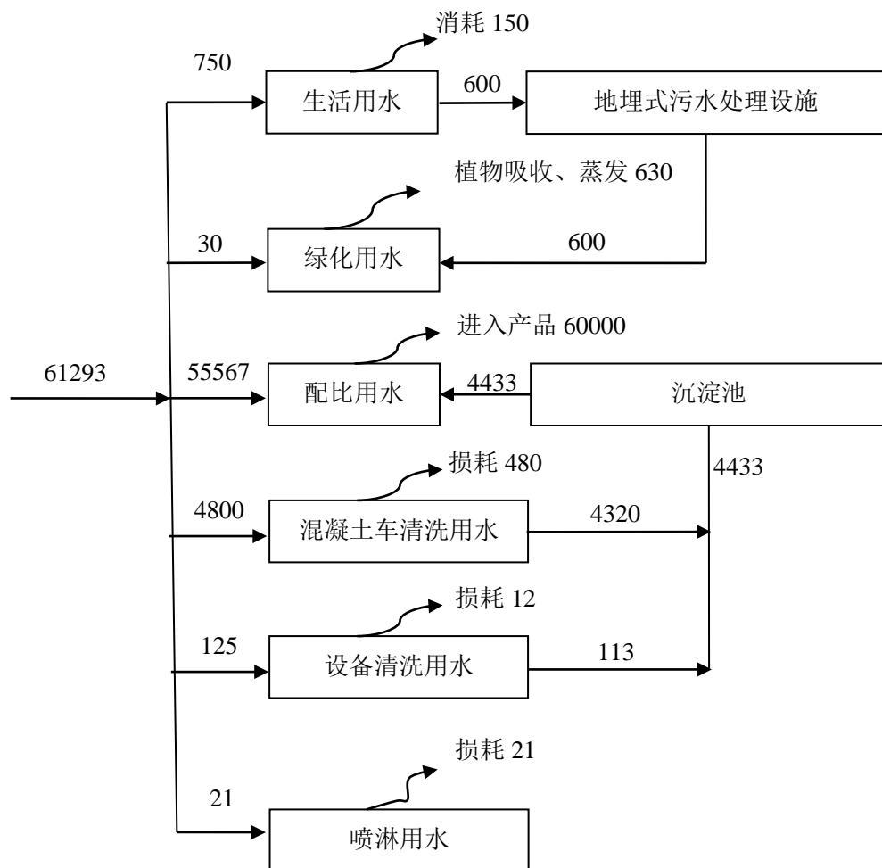
图 5-2 本项目用排水平衡图 t/a
