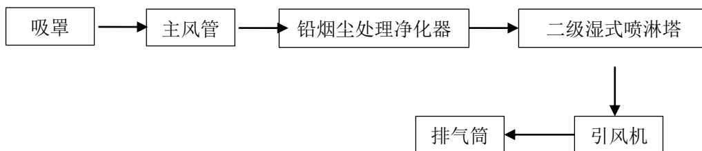
图 5-1 铅烟净化器工艺流程图
