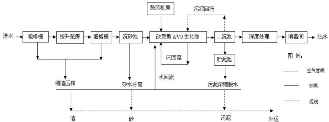
图 7-1 沭阳南方水务有限公司污水处理工艺流程图
