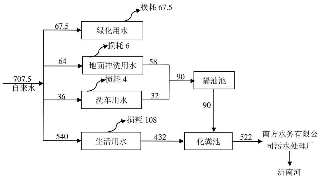
图 5-4 全厂平衡图（单位：t/a）
