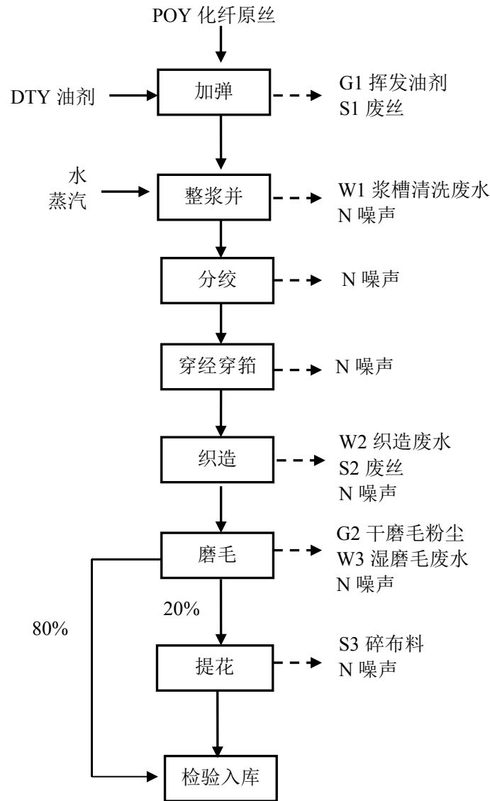
图 5-1 营运期生产工艺流程
