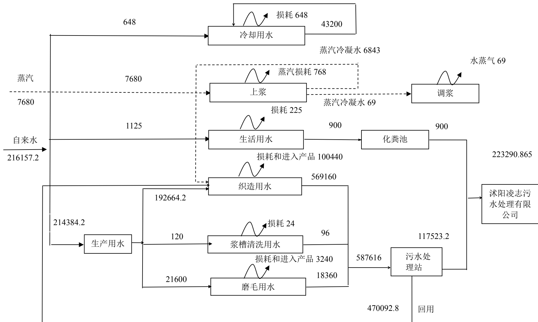
图 5-2 本项目水平衡图 (t/a)
