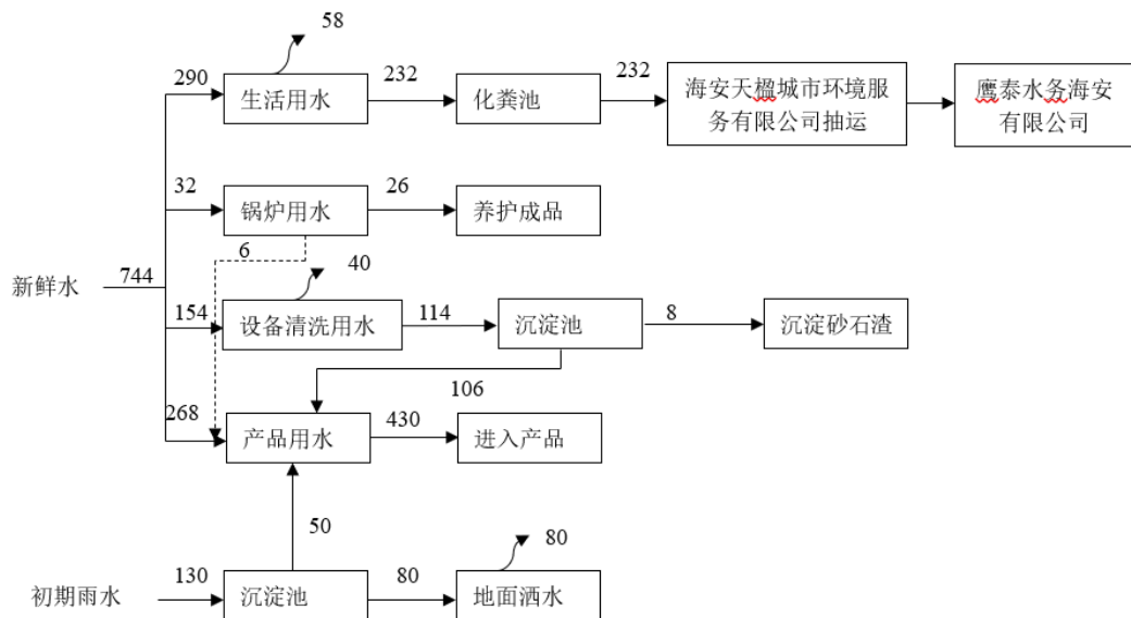
图 3-2 现有项目水平衡图（单位： \text{m}^3/\text{a} ）
