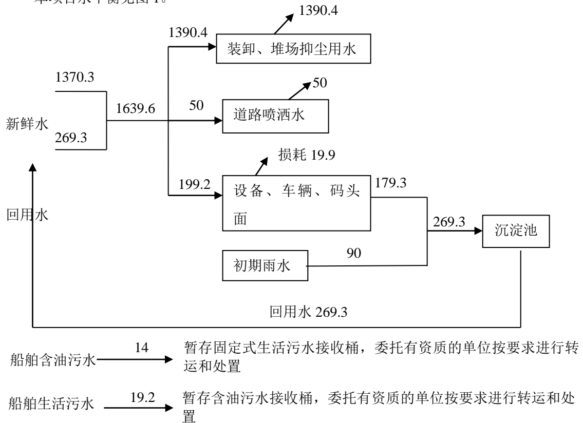
图 1 本项目水平衡图 t/a
