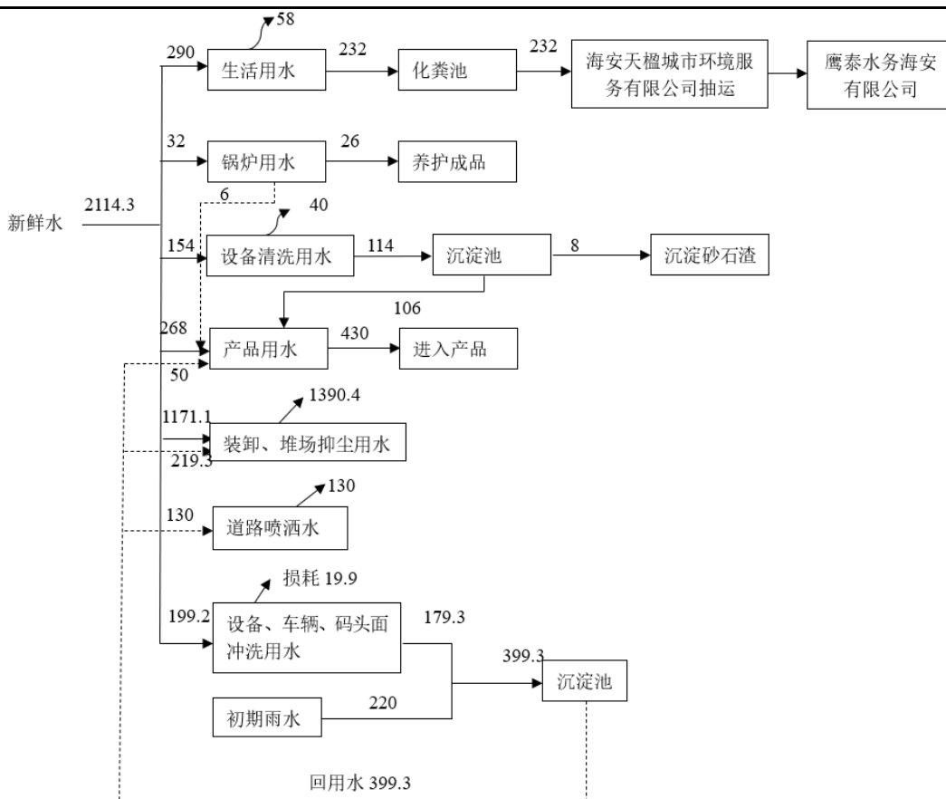
图 2 全厂水平衡图 t/a
