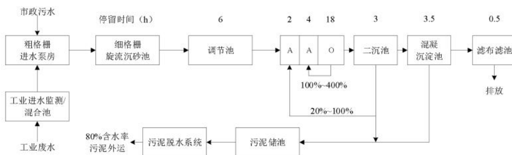
老坝港滨海新区污水处理厂污水处理工艺流程图
