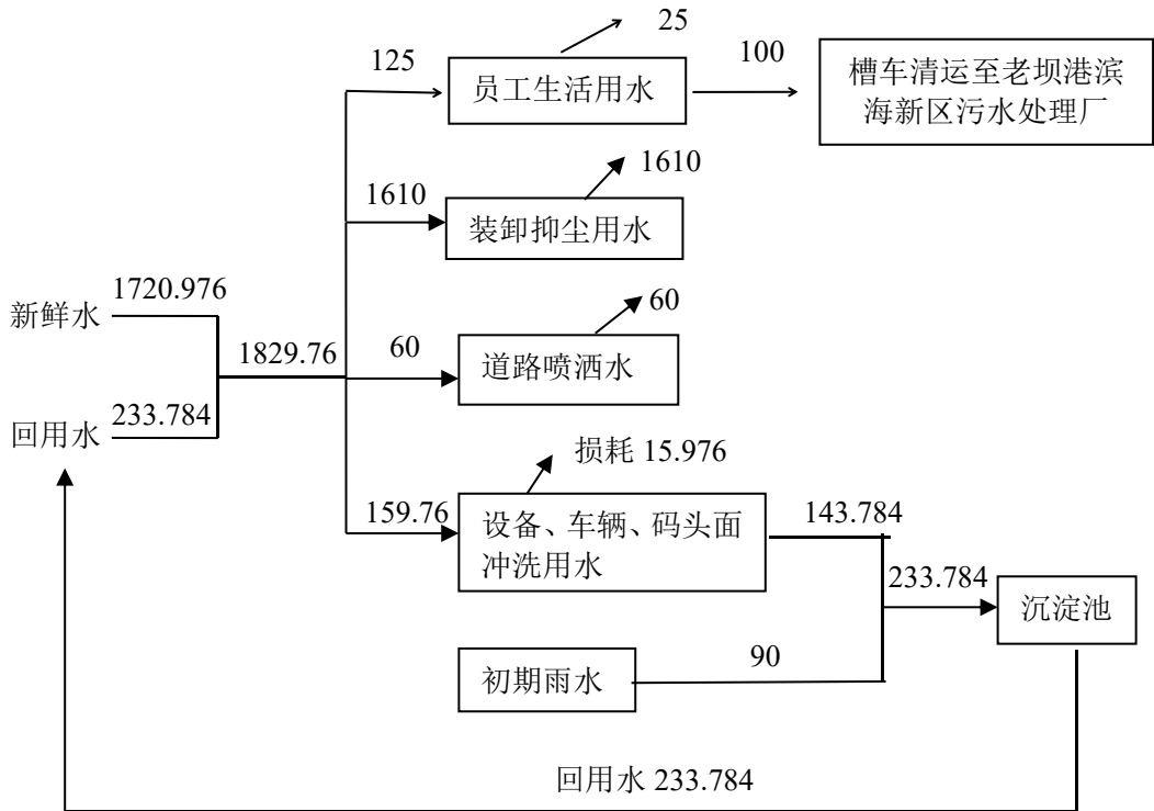
图 4-1 本项目水平衡图 t/a
