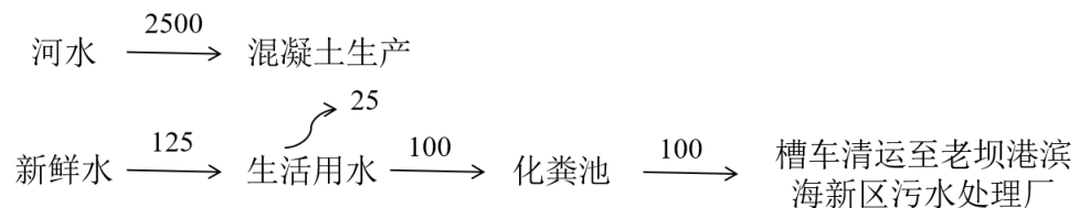
图 3-2 现有项目水平衡图 (单位: \text{m}^3/\text{a} )
