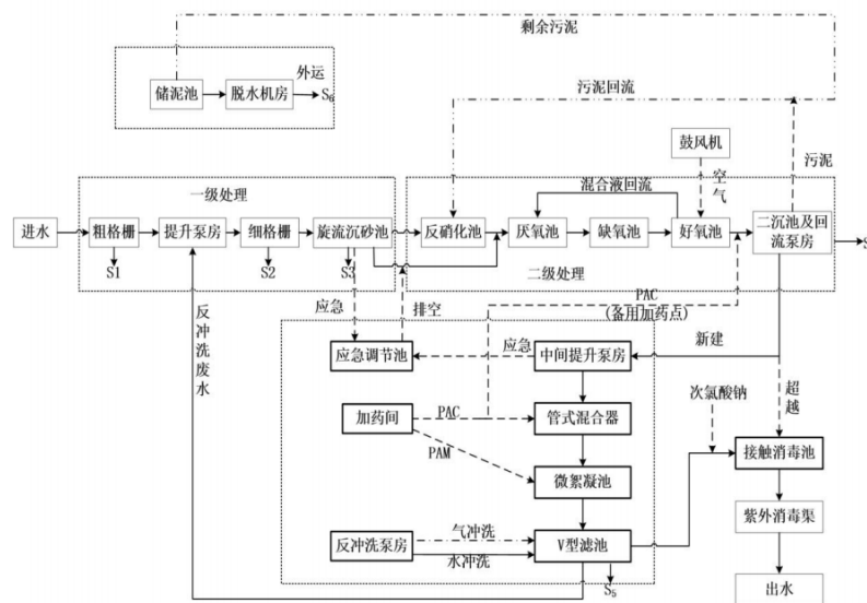
图 5-1 海安曲塘滇池水务有限公司工艺流程图
